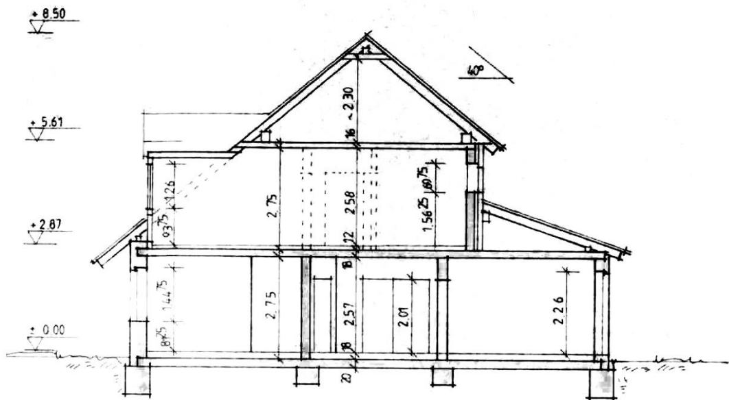
SCHNITT WOHNHAUS
