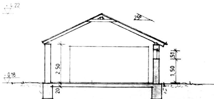
SCHNITT GARAGE
