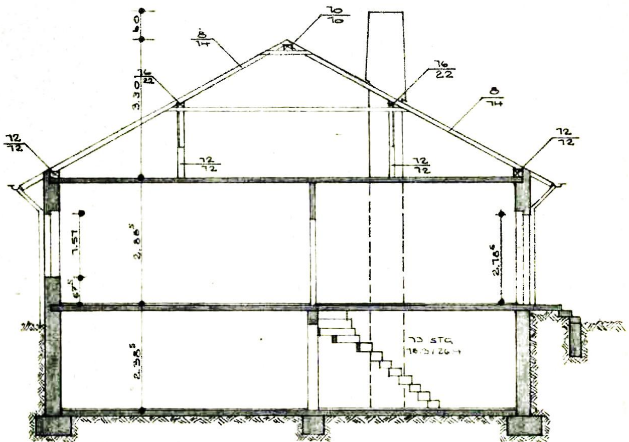
SCHNITT A-B
